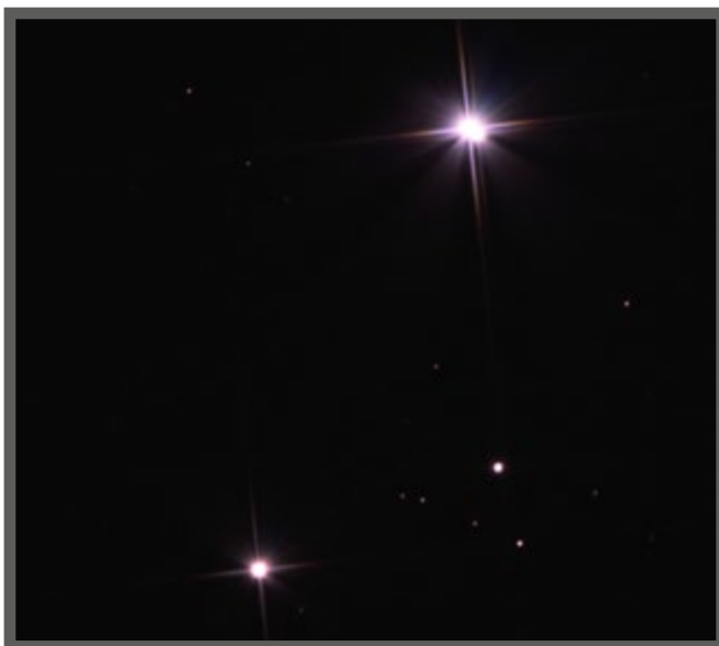
En esta fotografía podemos observar el sistema binario eclipsante "21 CEFE0"
